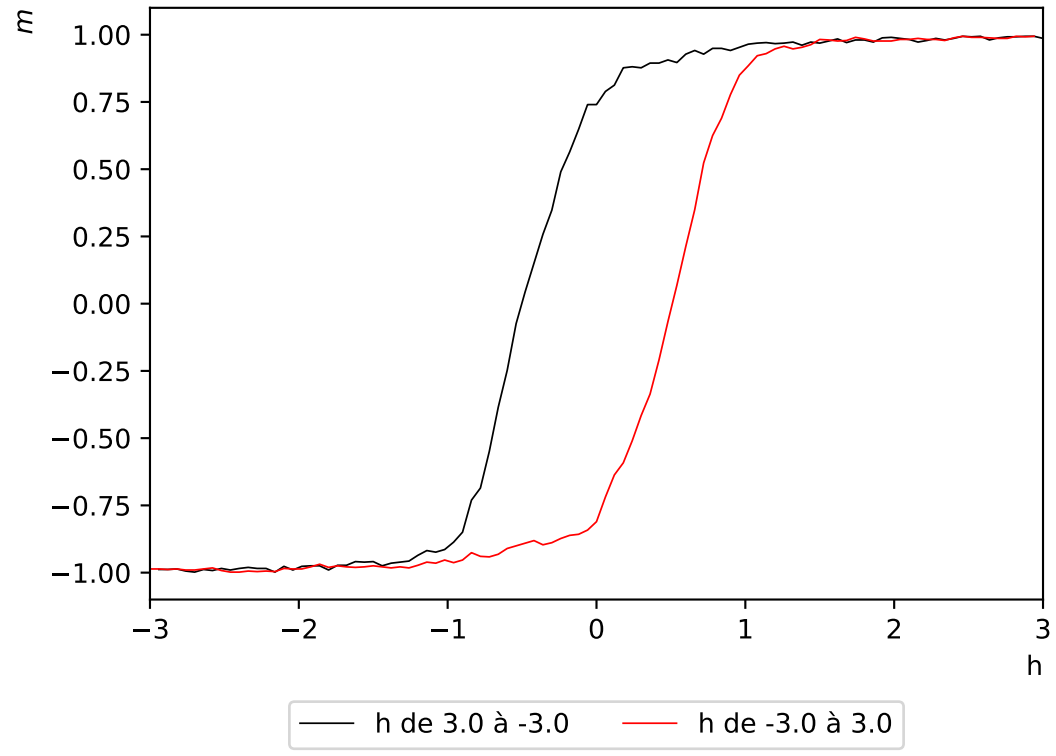
Hystérésis de l'aimantation - réseau de taille L=32 - champ magnétique d'amplitude h=3 à T=2.5
